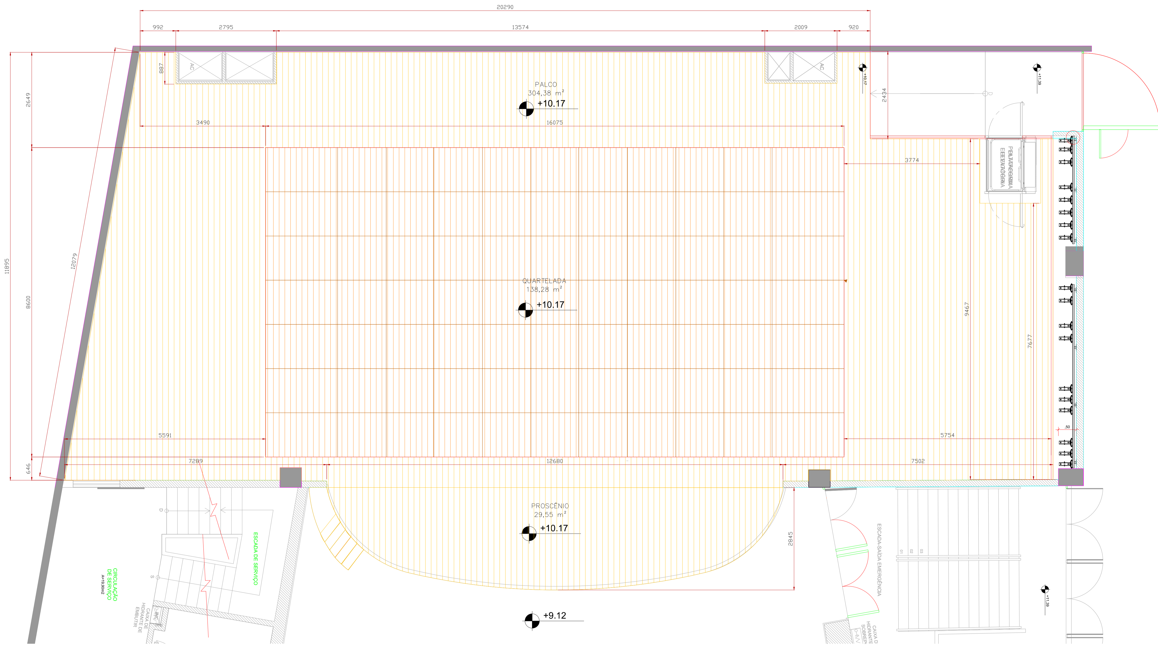
PLANTA BAIXA - PISO DO PALCO ESC. 1:50
